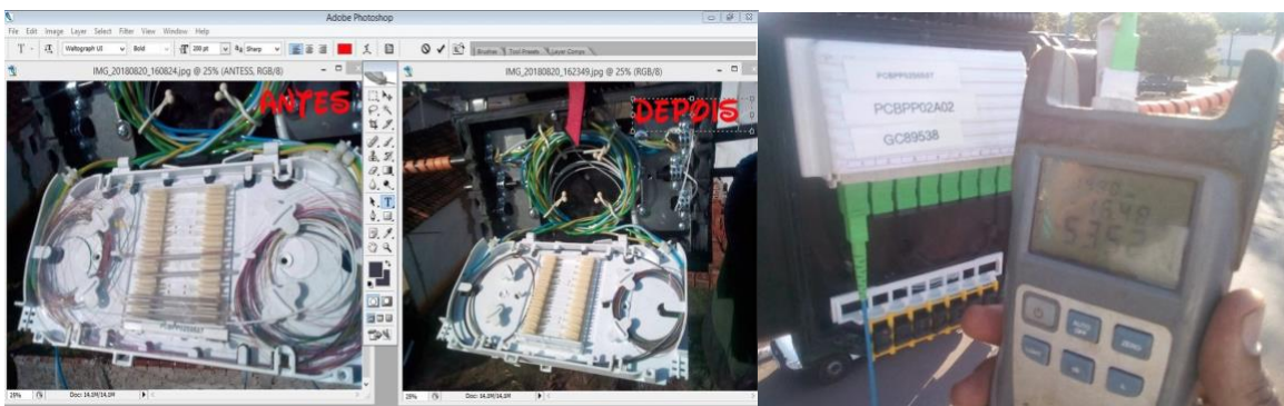
“NAP(C.T.O.) aérea 72Fo - com ATENUAÇÕES: Feito manutenção em 65 NAP(C.T.O.) corretiva e preventiva. Contrato: INOVAX engenharia de sistemas.
