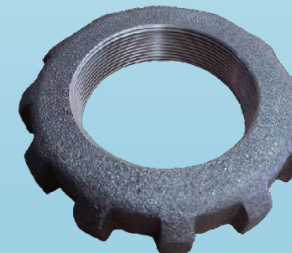
Porca do Eixo da Carreta Randon BSW 3.1/2" 13 FPP
