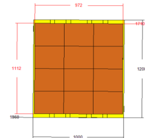
Vista superior
