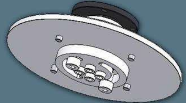
Limitador de rotación de 110 grados para binoculares DFN1 y DFN2 y los telescopios DFNT1 y DFNT2.
