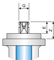
Detail 1 (D1) / Detalle 1 Front view / Vista frontal Connection / Conexión ISO 5211
