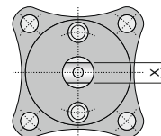
Detail 1 (D1) / Detalle 1 Top view / Vista superior Connection / Conexión ISO 5211
