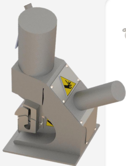
Proteção NR 12 Grampeadora
