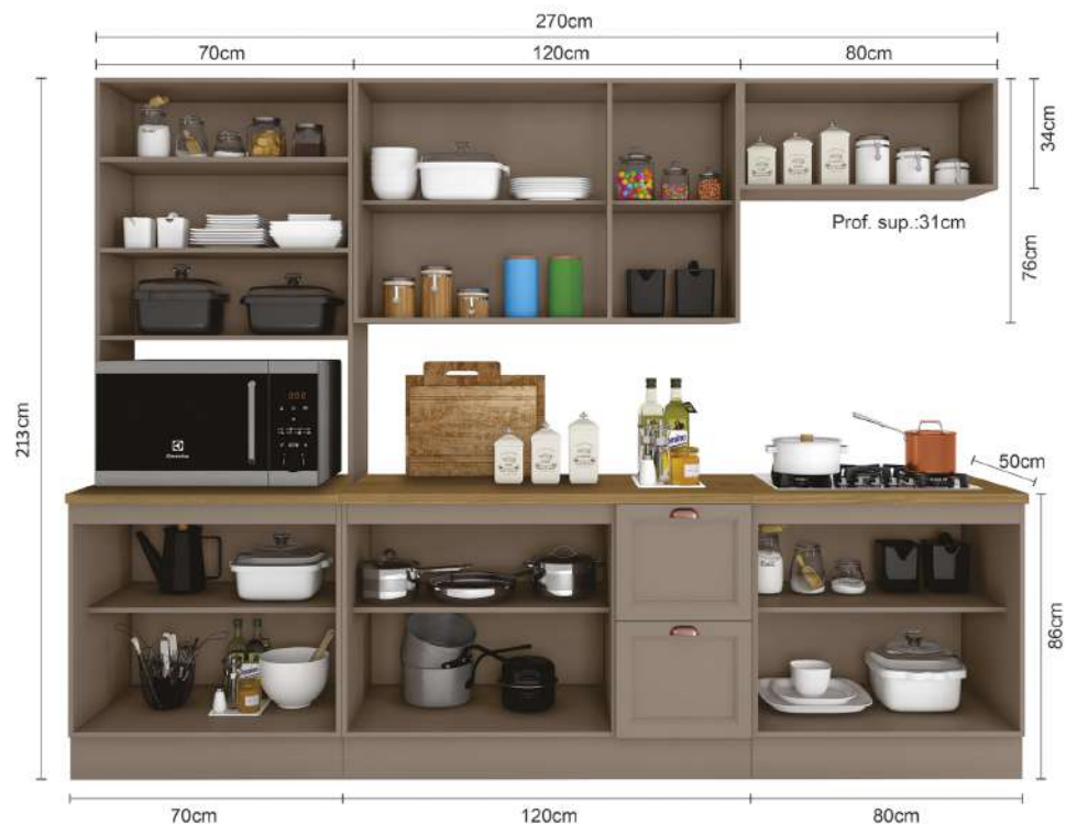
Rodapés Removíveis Modelo Click Removable click baseboards Zócalos de clic extraíbles
