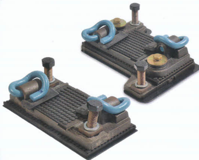
Conjuntos completos especiais para fixação de via permanente Elastic fixing set
