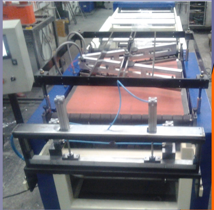
SELLADORA DE CAPUCHONES PARA FLORES
