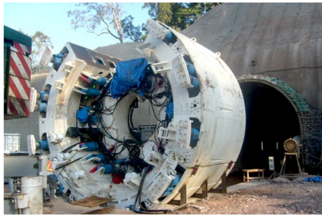
Proyecto hidroeléctrico Theun Hinboun Laos
