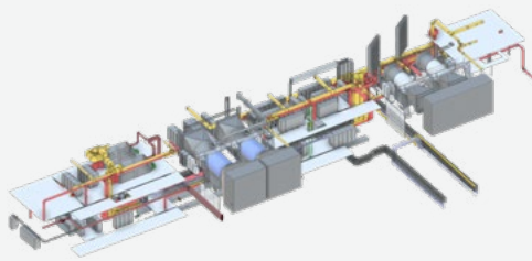
Sistema de ventilación de túnel carretero del San Gotardo Suiza
