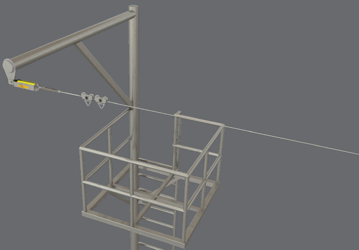
Diseño de estructuras y descarpaderos.
