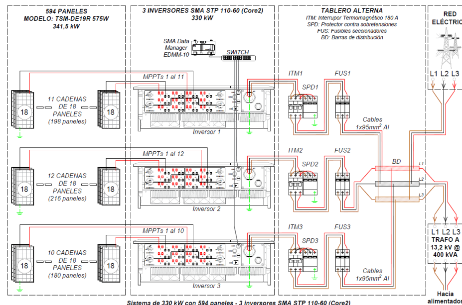
Sistema de 330 kW con 594 paneles - 3 inversores SMA STP 110-60 (Core2)
