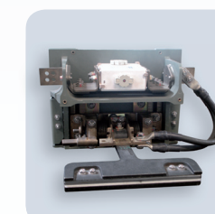
Captadores de corriente 3º carril, contacto superior
