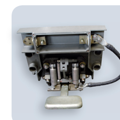
Captadores de corriente 3º carril, contacto inferior
