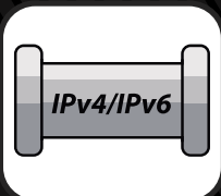
IPv4/ IPv6
