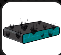
DDoS
