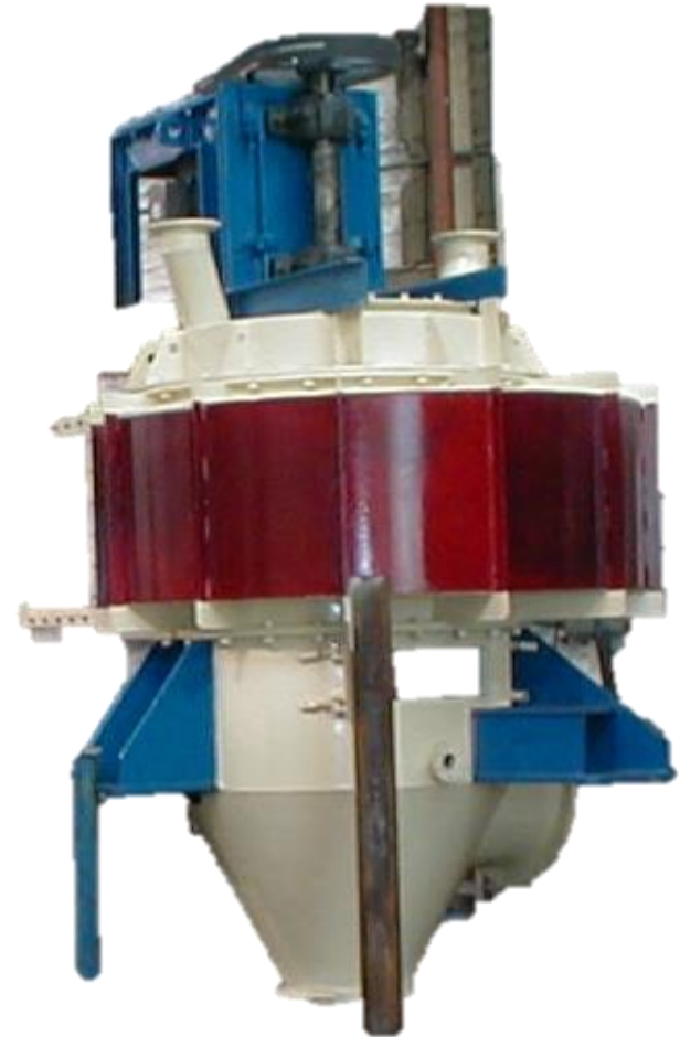
Clasificadores dinámicos
